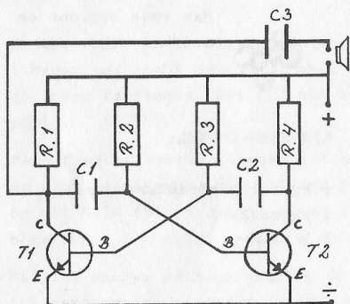
fig. 1. Diagram af Morsesummeren.
