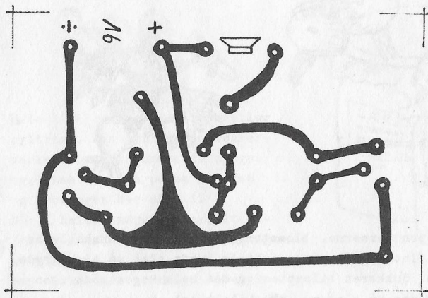
Fig. 2. Printpladen set fra Kobbersiden.
